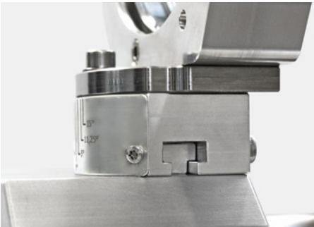
Horizontale und vertikale Verstellung
